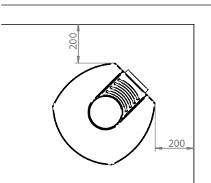
Abstand zu brennbarem Material ohne isoliertem Rauchrohr
